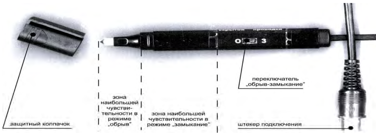
Рисунок 5.3.4.1 – Мини-датчик МД-01
