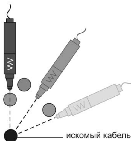
Рисунок 5.4.2 – Поиск кабеля (жилы) по минимуму сигнала
