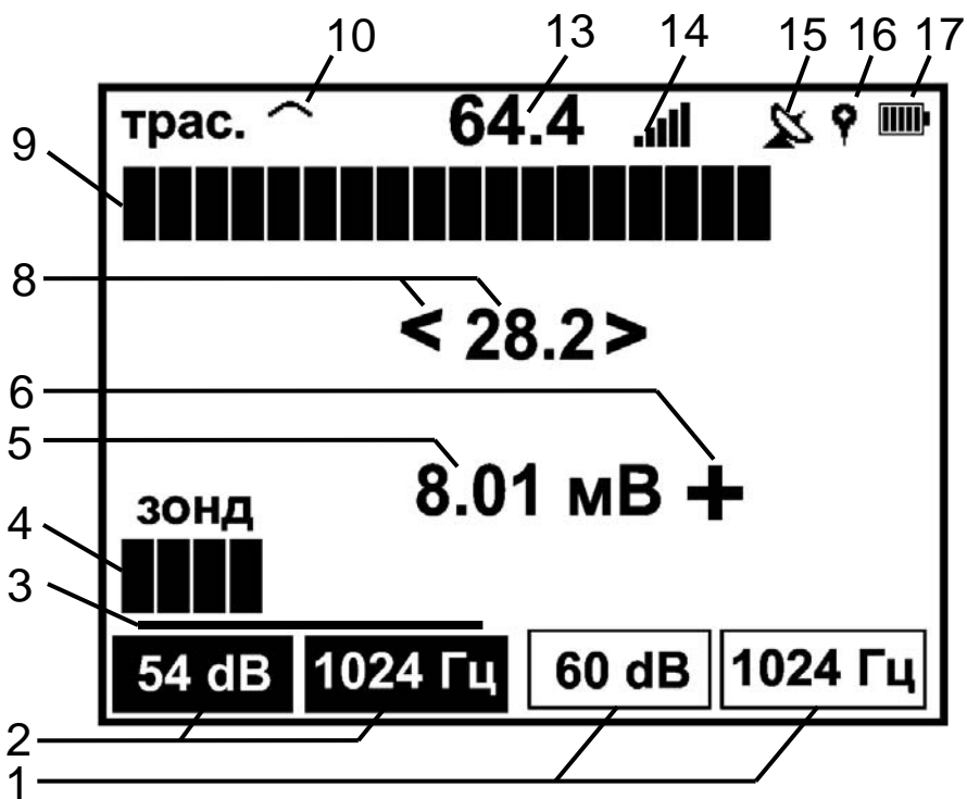
Рисунок 3.4 – Индикатор в режиме «ТРАССА» (а) и «ТРАССА-ЗОНД» (б)
